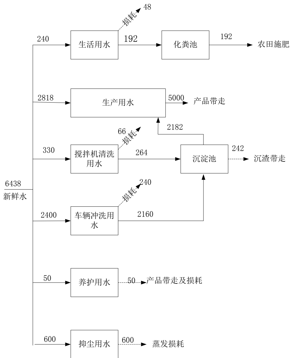
图2-1 项目水平衡图 (单位m 3 /a)
