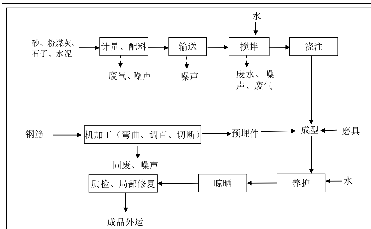
图二 生产工艺流程图
