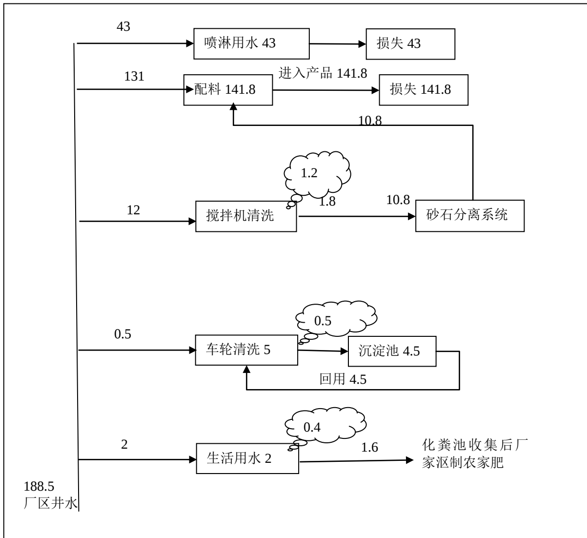
图三 本项目水量平衡图 (m³/d)
