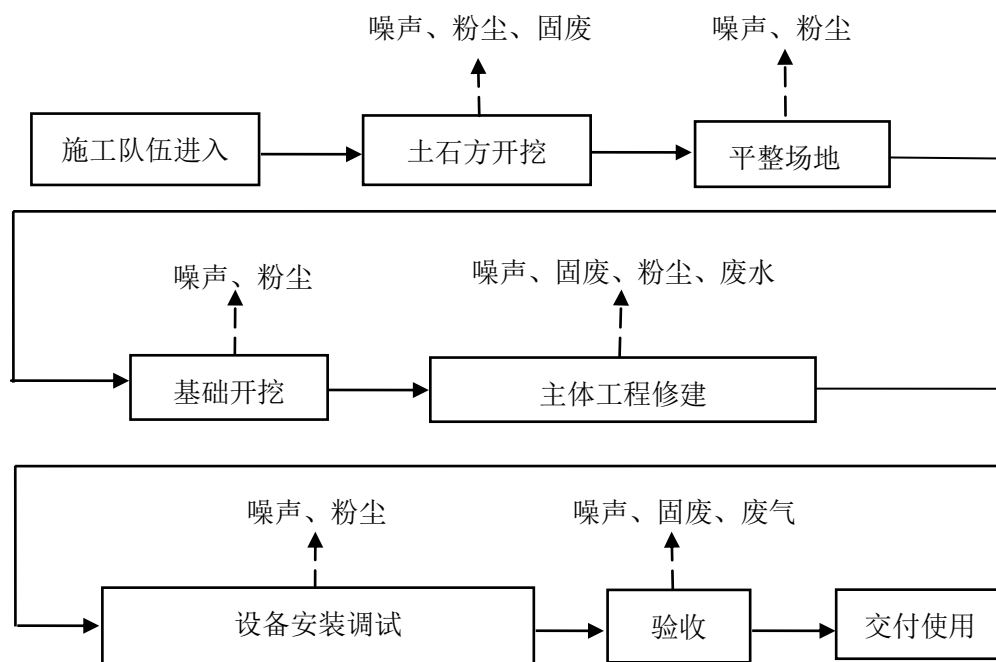
图一 本项目施工期工艺流程图
